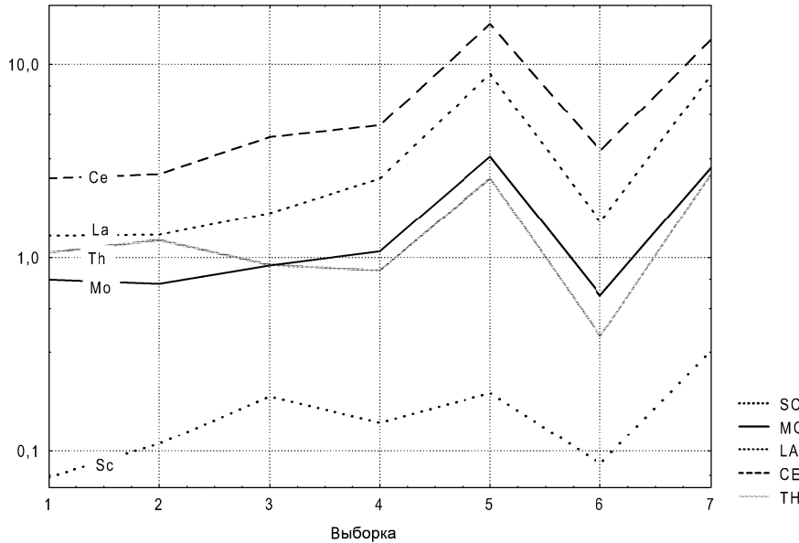
Рис. 3. Средние содержания (г/т) скандия, молибдена, лантана, церия и тория в кварцах из вулканитов ЭВЦ
