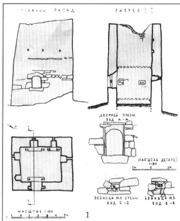
Рис. 2. 1 – Фасад, план и разрез боевой башни в с. Дзивгис. 2 – Скальная крепость «Дзывгъисы фидар». Фасад, план, разрез башни № 5. Обмер и чертеж С. А. Пирогова
