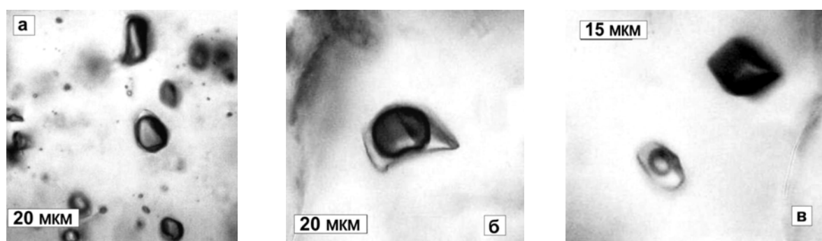
Рис. 3. Флюидные включения в минералах карбонатных ксенолитов а – газные и существенно газные ФВ (V); б – водно-солевое ФВ (VL); в – сингенетическое водно-солевое (VL) и газное (V) ФВ.
