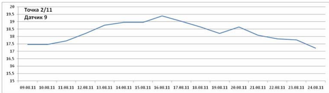
Рис. 4. График измерения температуры термодатчиком № 9
