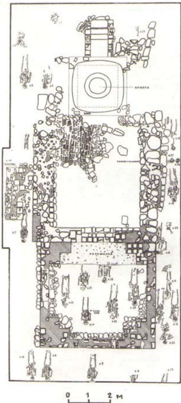
Рис. 3. План церкви № 2 и крипты (по В.А. Кузнецову, 2003)
